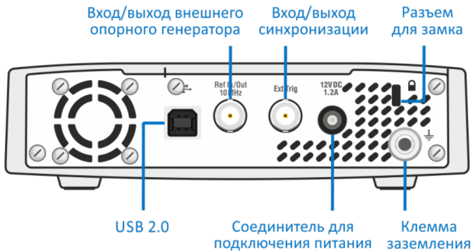
Рисунок 4.4 Задняя панель
