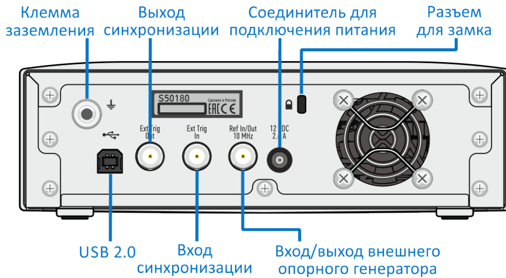
Рисунок 4.10 Задняя панель
