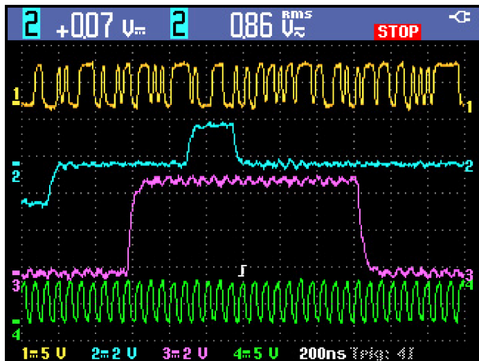
Четыре изолированных входных канала легко справляются со смешанными сигналами любого типа.
