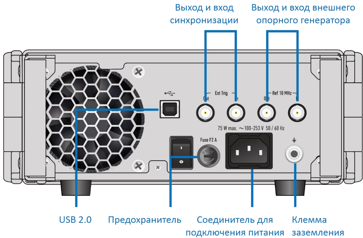
Рисунок 4.14 Задняя панель
