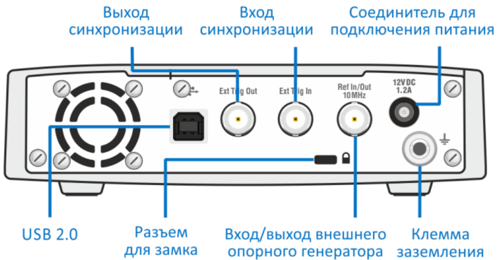
Рисунок 4.8 Задняя панель
