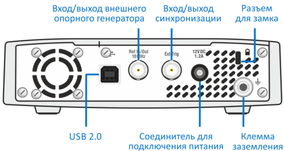
Рисунок 4.4 Задняя панель
