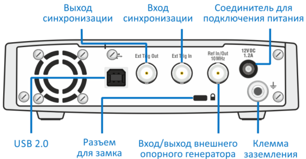
Рисунок 4.2 Задняя панель
