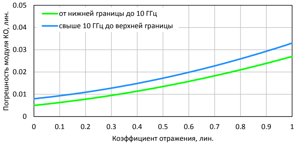
Погрешность измерений модуля коэффициента отражения анализаторов S5045, S5048, S5065, S5085, S50180, S7530
