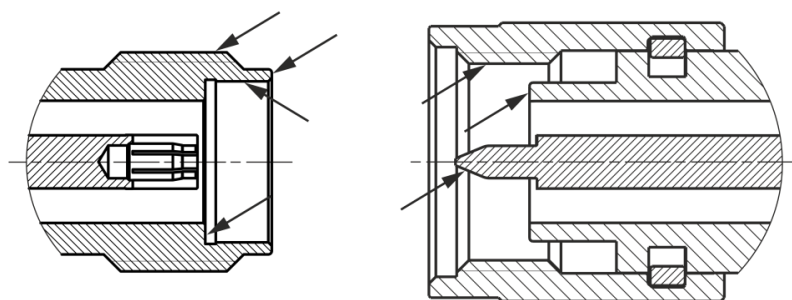
Рисунок 3.2 Соединители тип 2,4 мм (розетка и вилка)
