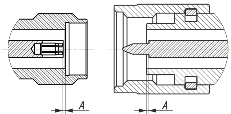
Рисунок 3.4 Соединители тип 2,4 мм (розетка и вилка)
