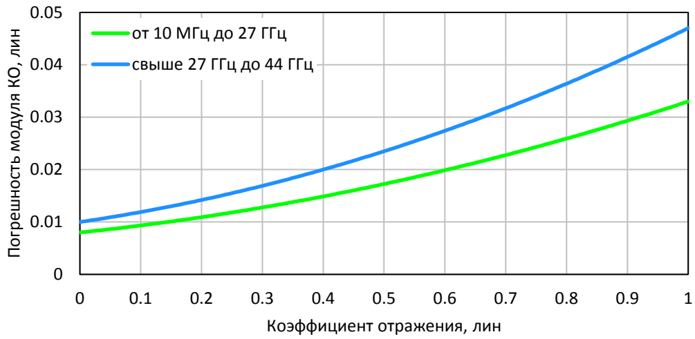
Погрешность измерений модуля коэффициента отражения анализаторов S50244
