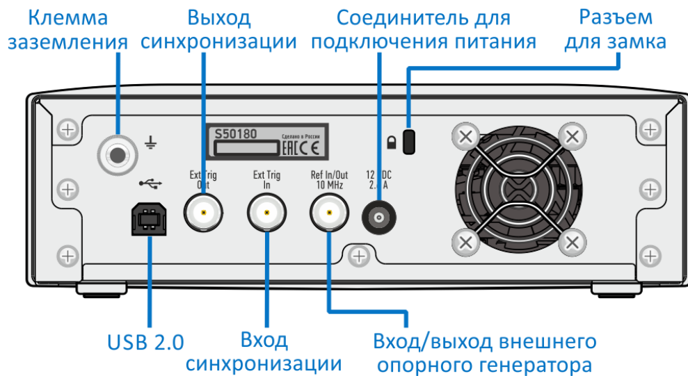
Рисунок 4.10 Задняя панель
