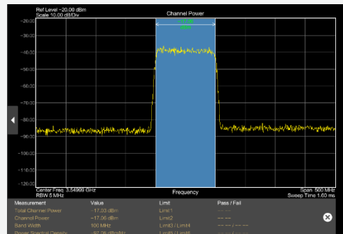
Измерение мощности в канале
