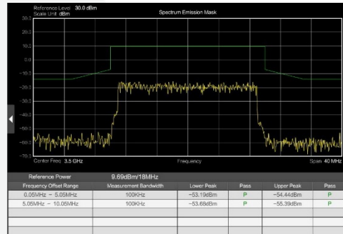
Спектральная маска излучения LTE/LTE-A
