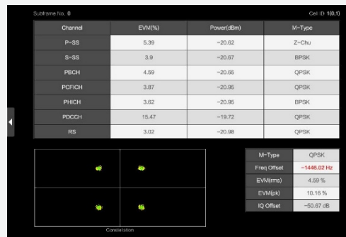
Канал управления LTE/LTE-A
